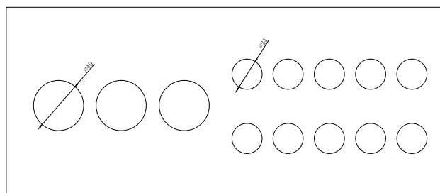
箱体底部开孔图
