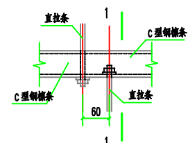
屋面直拉条安装节点
