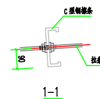
屋面直拉条、斜拉条及撑杆安装节点
