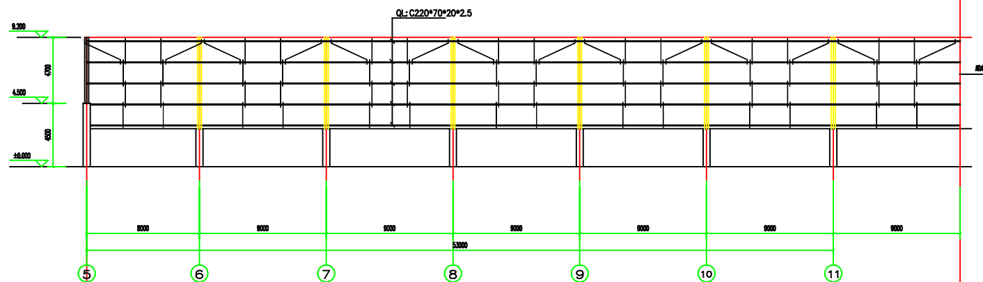
钢架布置图 1:150
