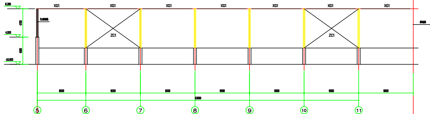
钢架布置图 1:150
