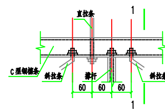
屋面直拉条、斜拉条及撑杆安装节点
